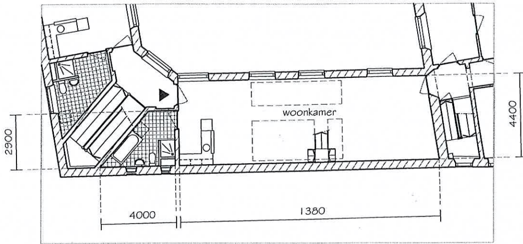
eerste verdieping
